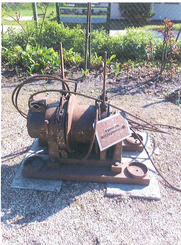
Sujtólégbiztos vitla felújítás előtt
